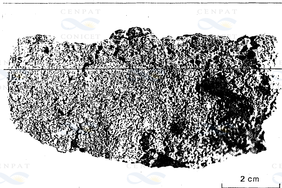
Figura 22: Horizonte vesicular, clase 4 de condición superficial. PS, parte superior y PI, parte inferior.
