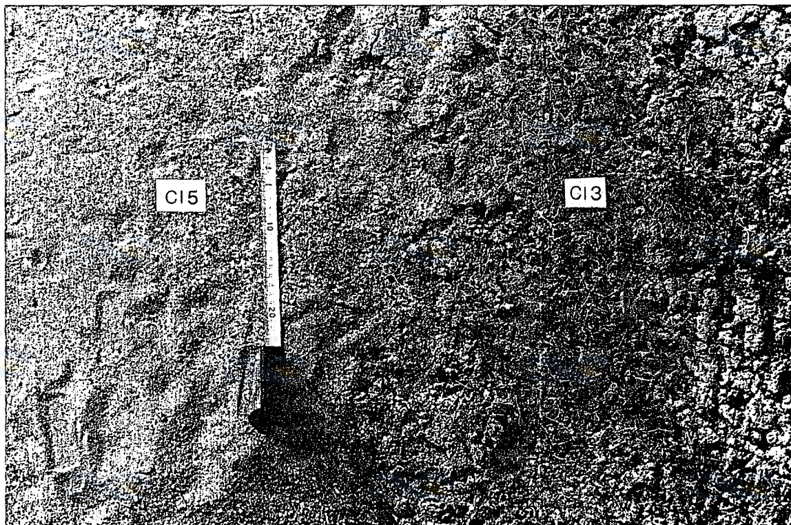
Figura 17: a) Clase 3 de condición superficial. Destrucción de agregados y hundimiento de gravas durante la estación fría. En este caso la clase 3 (Cl 3) limita con la clase 5 de acumulación arenosa (Cl 5). b) Depresiones alrededor de gravas (D).
