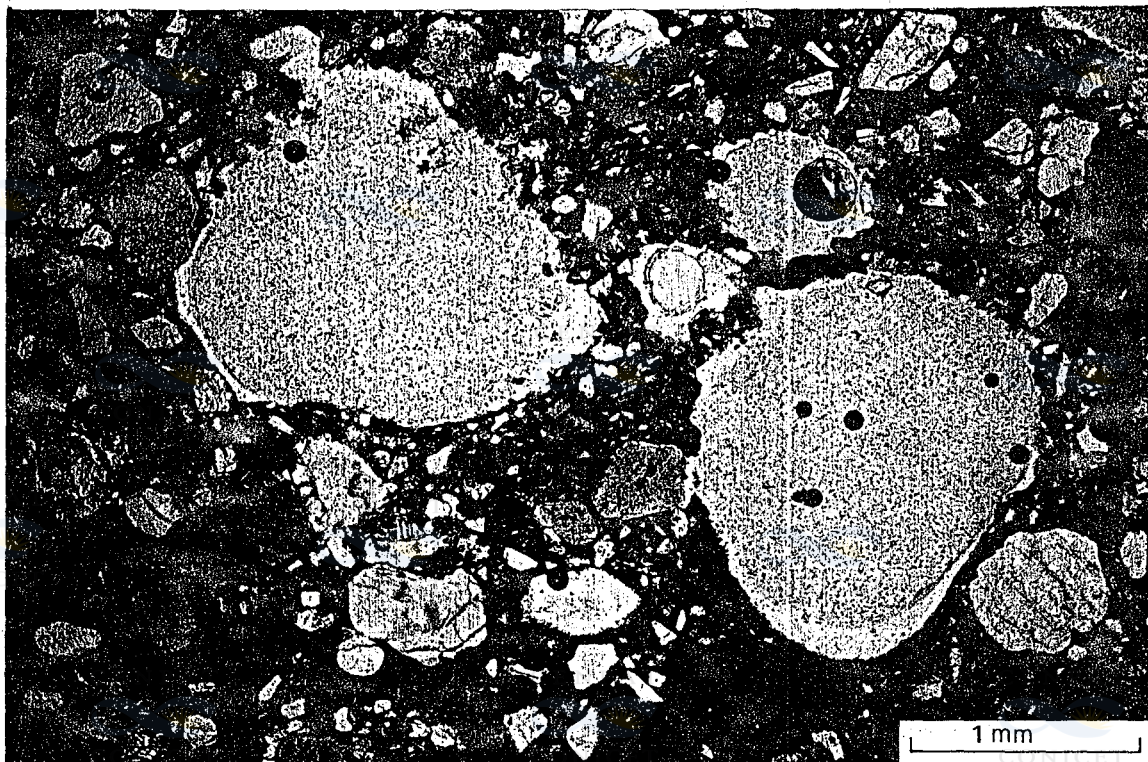
Figuras 28 y 29: Microfotografías de la costra estructural vesicular (horizonte Av); parte superior. Estructura vesicular entre granos. Vesículas equidimensionales, con paredes lisas en la base e irregulares en el techo. X 25, luz normal.
