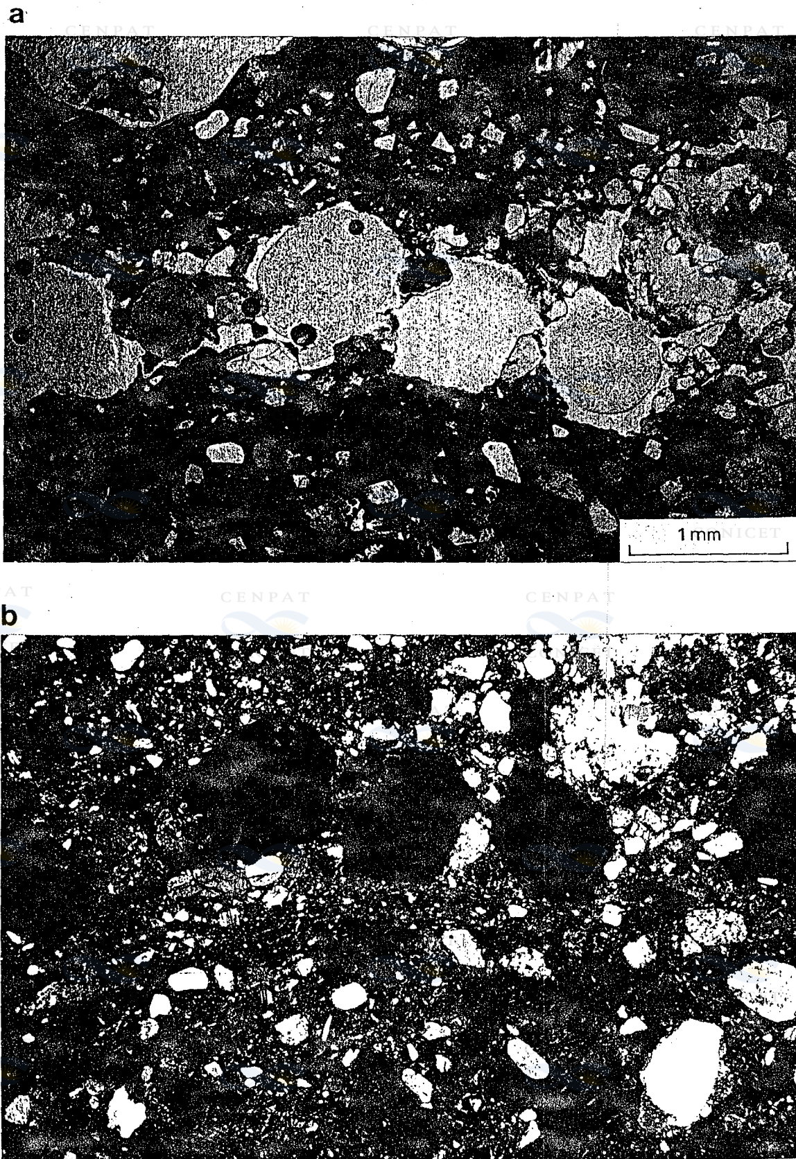
Figura 30: Microfotografías de la costra estructural vesicular. Obsérvese el aumento del espacio poral por la coalescencia de vesículas equidimensionales. X 25, a) luz normal; b) nicoles cruzados; la fábrica-b del material fino es en motas aisladas.
