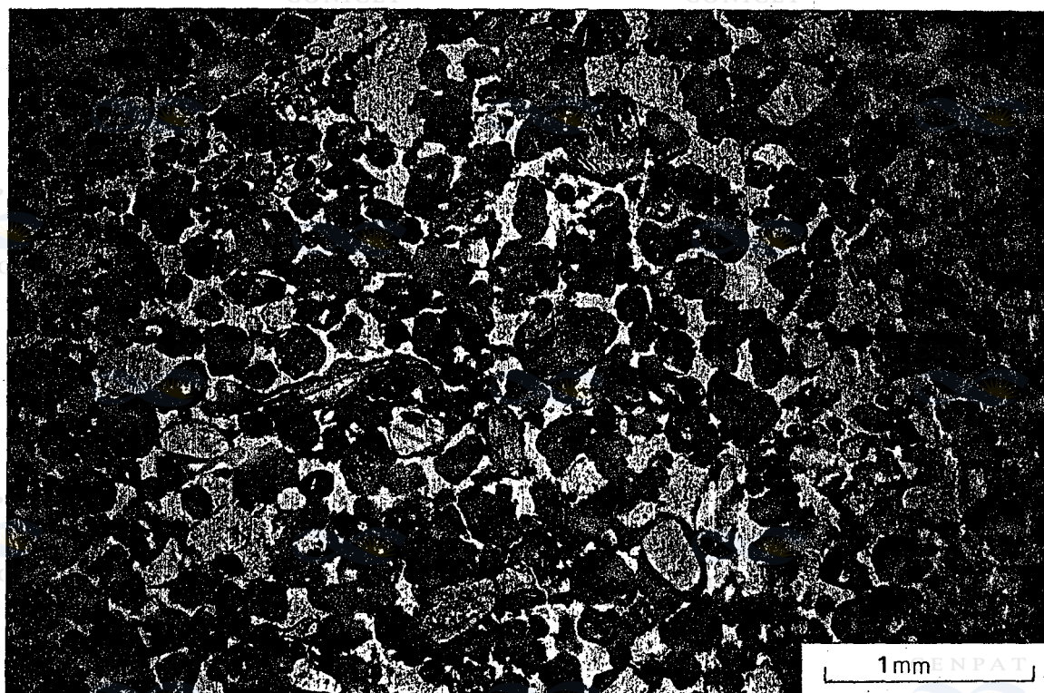
Figura 42: Microfotografía del horizonte argílico de estructura granular en contacto con el horizonte 2Btk de estructura en bloques angulares mal definidos y fisurada. La fábrica-b del material fino es en motas aisladas y en mosaicos. X 25, a) luz normal; b) nicoles cruzados.
