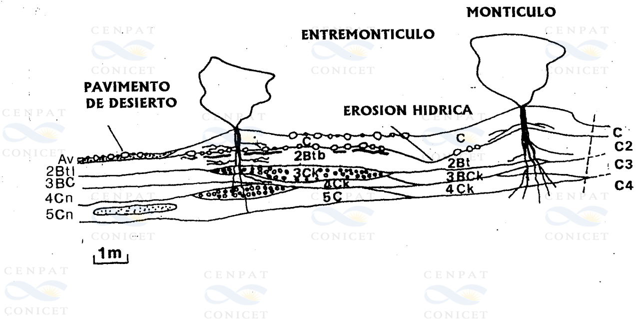
Figura 4: Esquema de una sección transversal de los suelos y del microrelieve en el Bajo de la Suerte (adaptado de Súnico et al., 1993).
