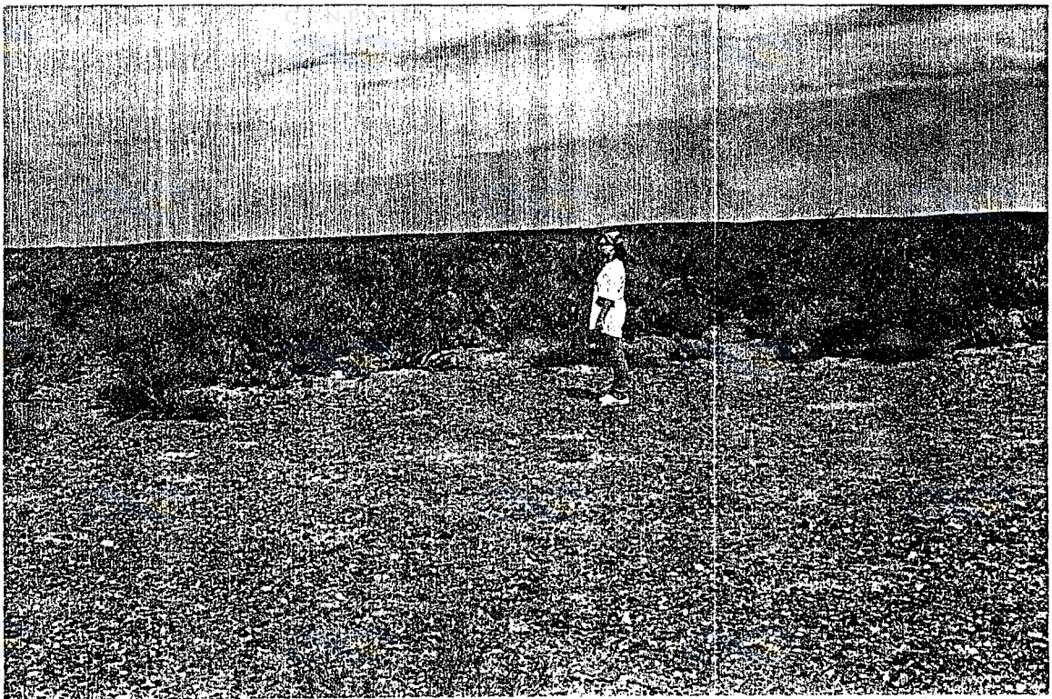
Figura 19: Pavimento de desierto de mayor extensión. Obsérvese los fragmentos de tamaño piedra que se encuentran sueltos en superficie.
