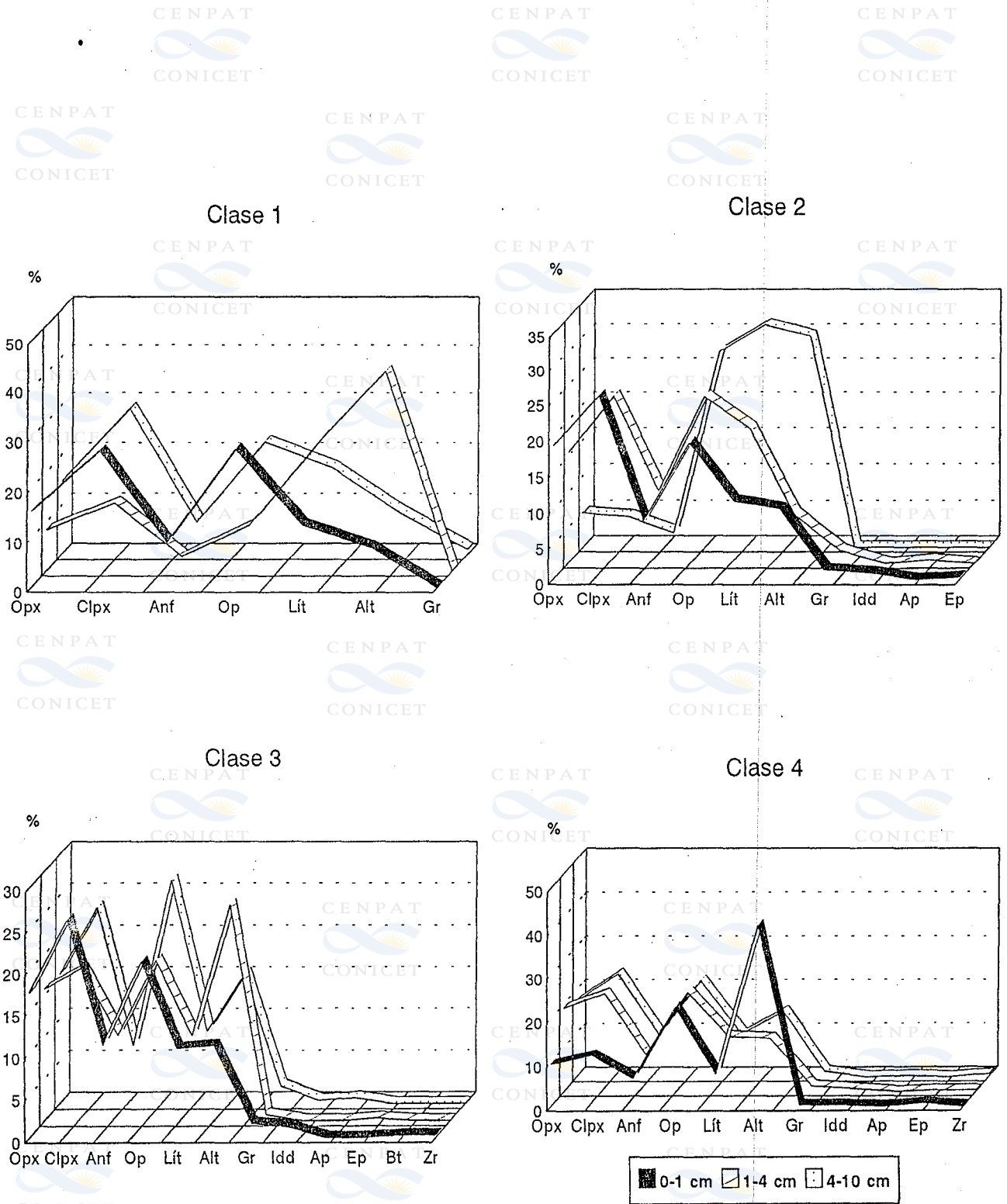
Figura 57b: Distribución porcentual de las especies minerales pesadas. Bajo de la Suerte, clases de condiciones superficiales.
