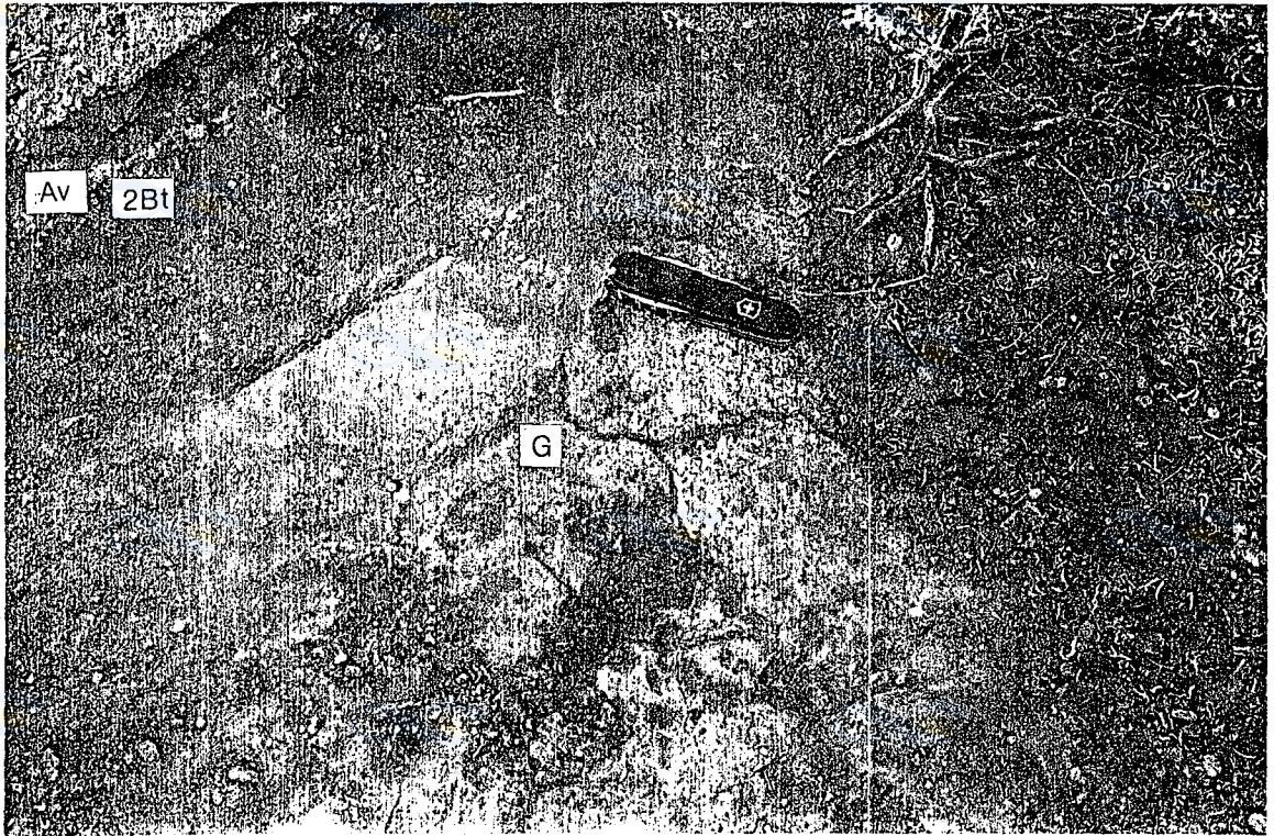
Figura 15: Detalle del límite superior del horizonte 2Bt con signos de erosión hídrica encauzada.
